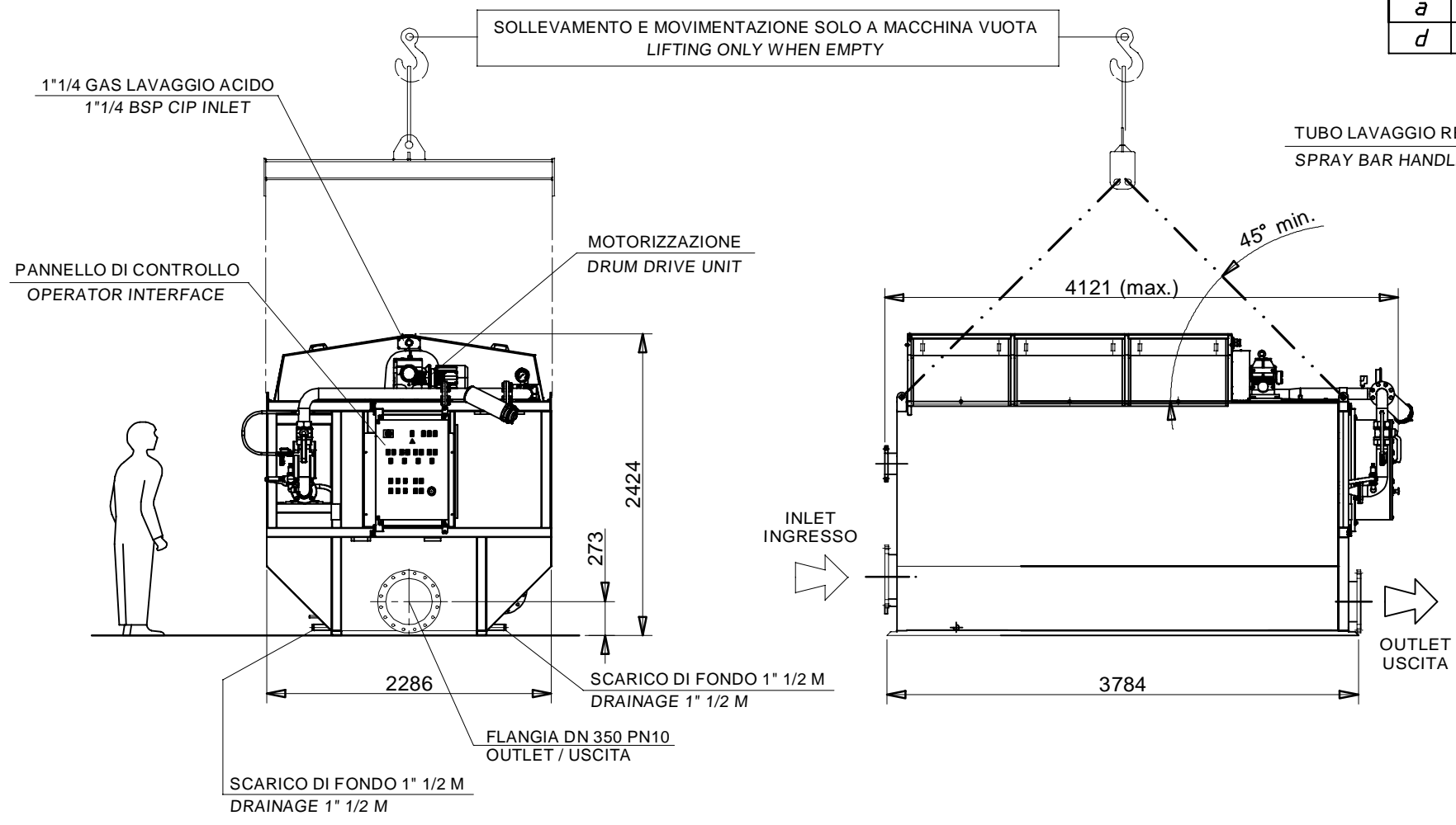
DIMENSIONI DI MASSIMO PER IL TRASPORTO MAXIMUM TRANSPORT DIMENSIONS
