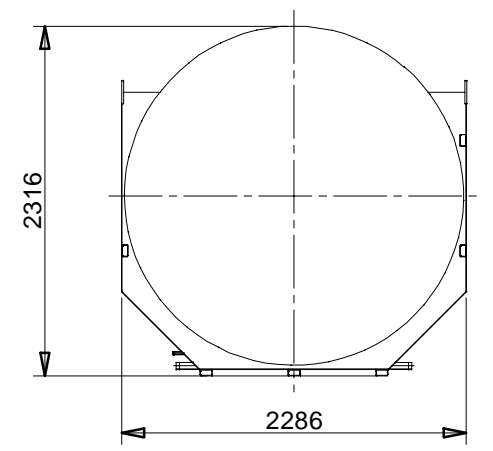
DIMENSIONI DI MASSIMO PER IL TRASPORTO MAXIMUM TRANSPORT DIMENSIONS
