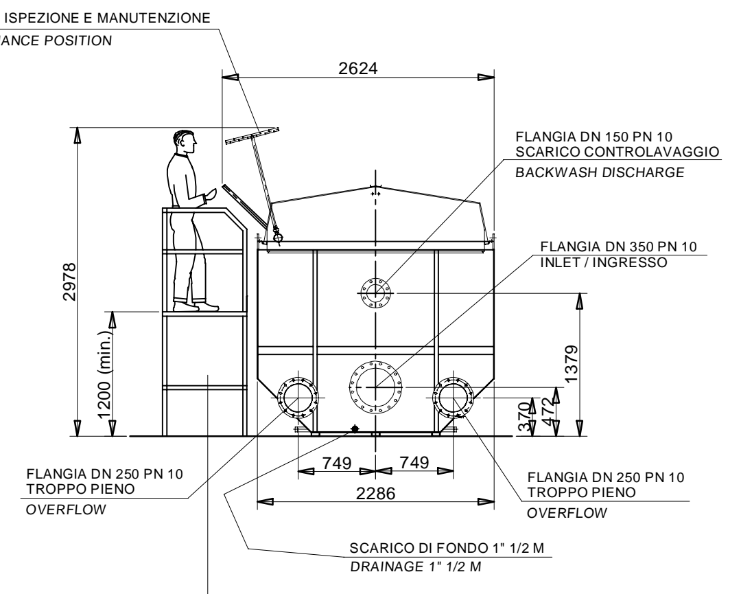
PIATTAFORMA CONSIGLIATA PER ISPEZIONE E MANUTENZIONE (NON FORNITA) SUGGESTED PLATFORM FOR INSPECTION AND MAINTENANCE (NOT SUPPLIED)
