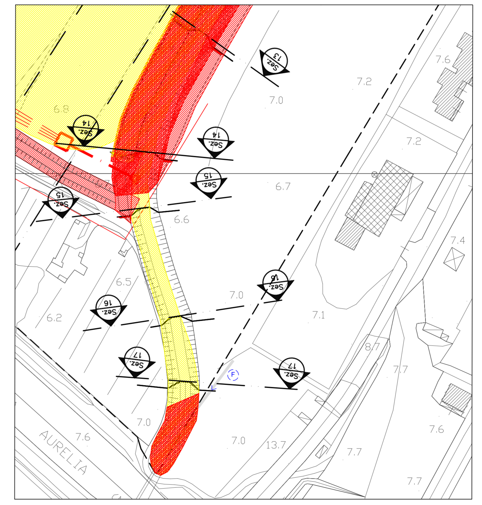
PLANIMETRIA Scala 1:1.000
