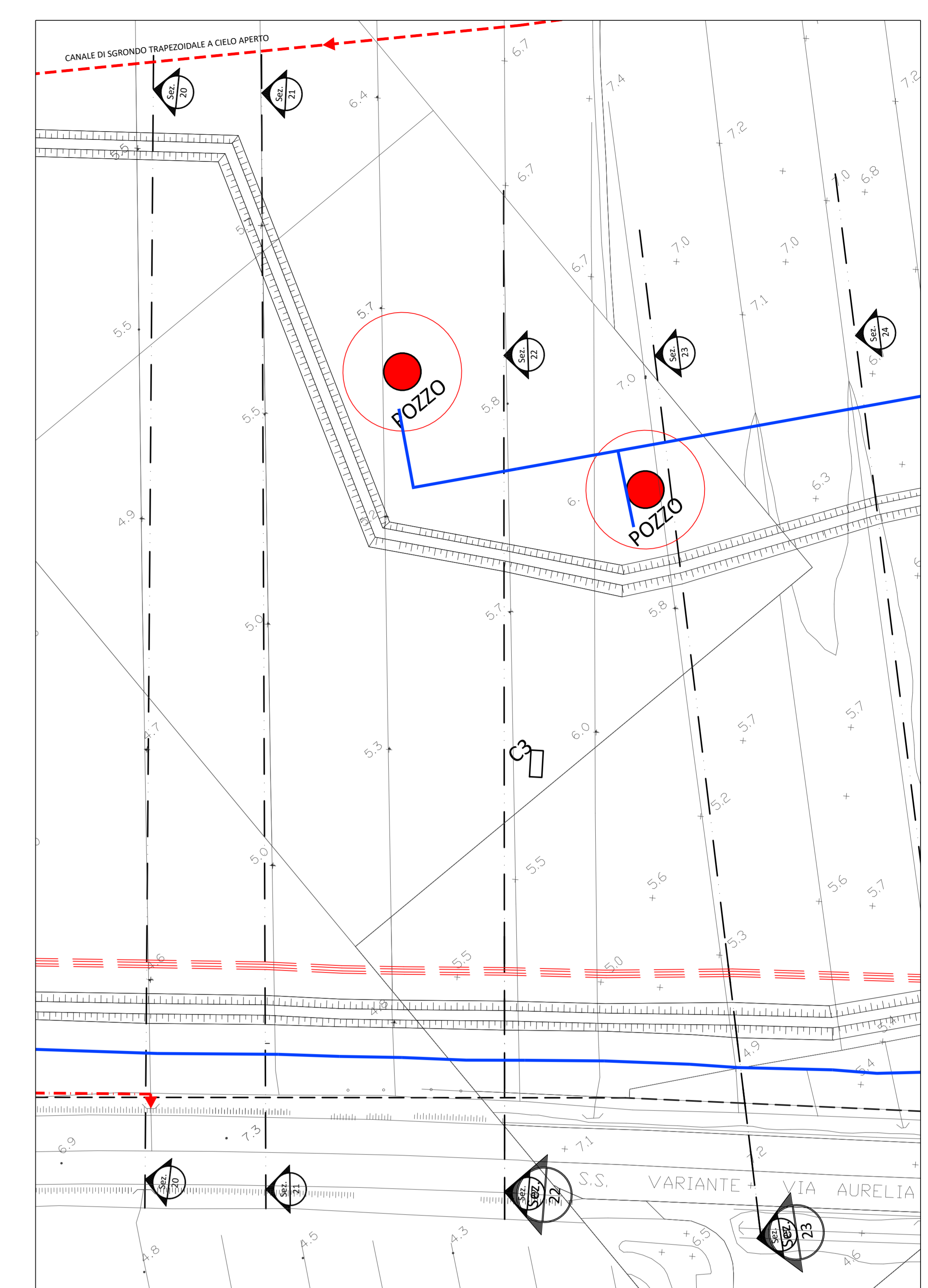
PLANIMETRIA Scala 1:1.000
