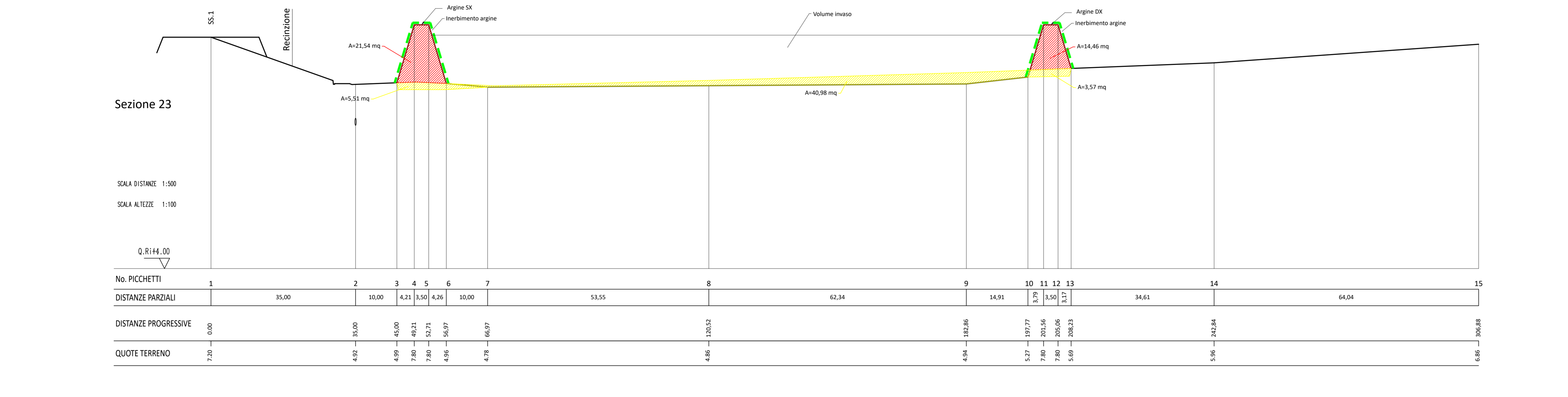
SEZIONE 23 Scala 1:500/100
