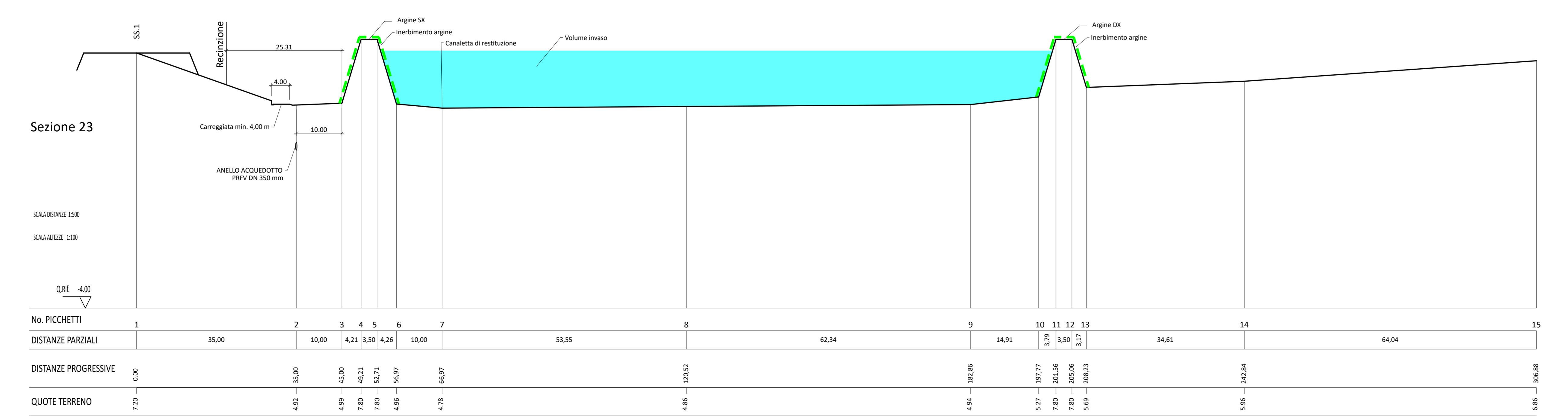
SEZIONE 23 Scala 1:500/100
