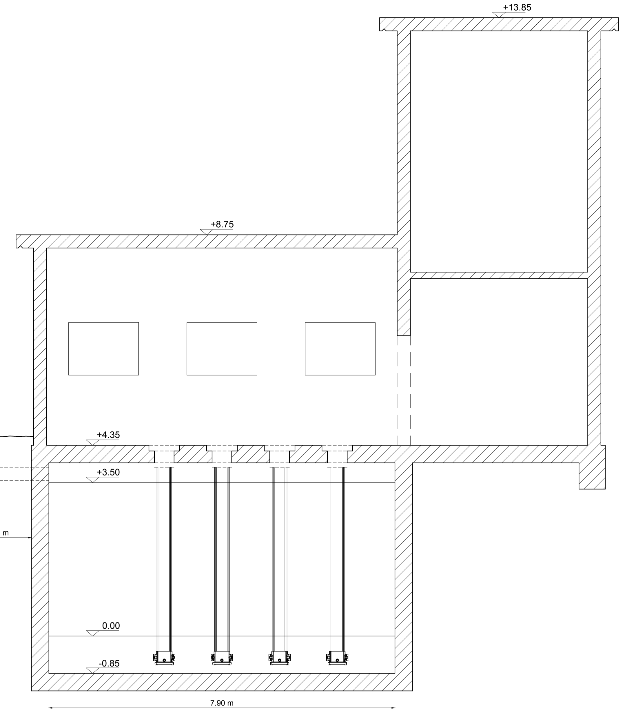
Sezione B - B
