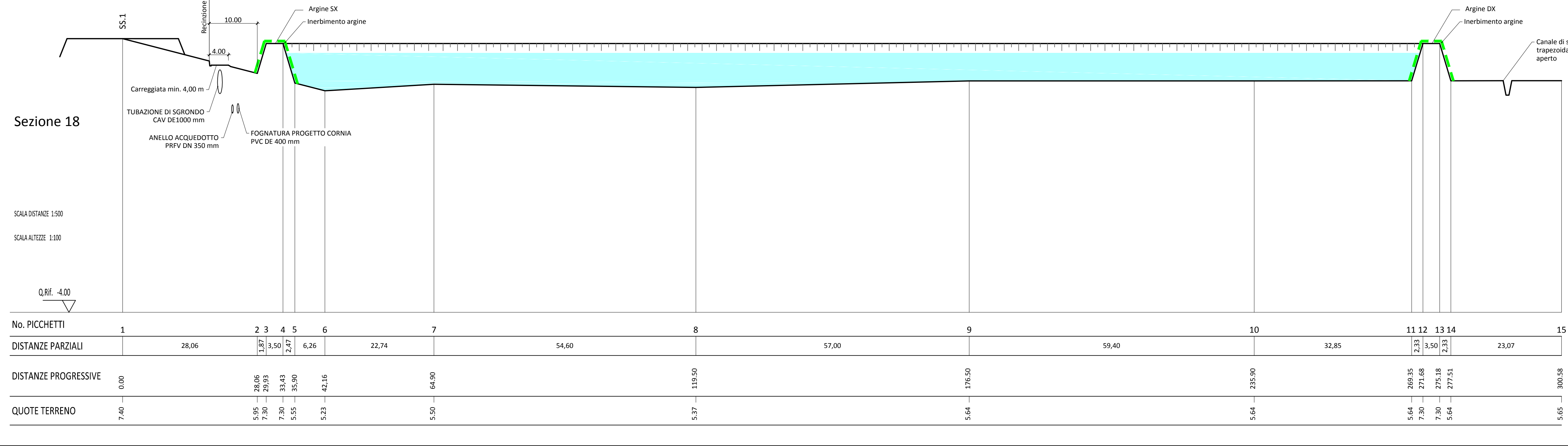
SEZIONE 18 Scala 1:500/100
